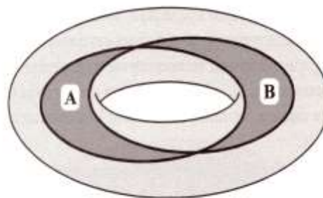
Figure XVII-22 différence symétrique tracée sur un tore
